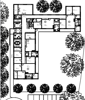
Vorentwurfsplanung Kindergarten
